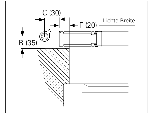
Montageart 4 aufliegend
