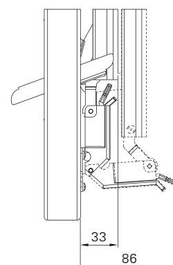
Verstellhebel
