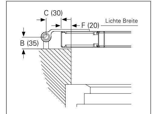
Montageart 4 aufliegend
