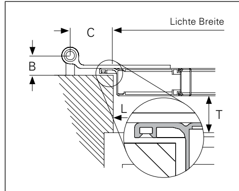
Montageart 2 stumpf mit Falzleiste
