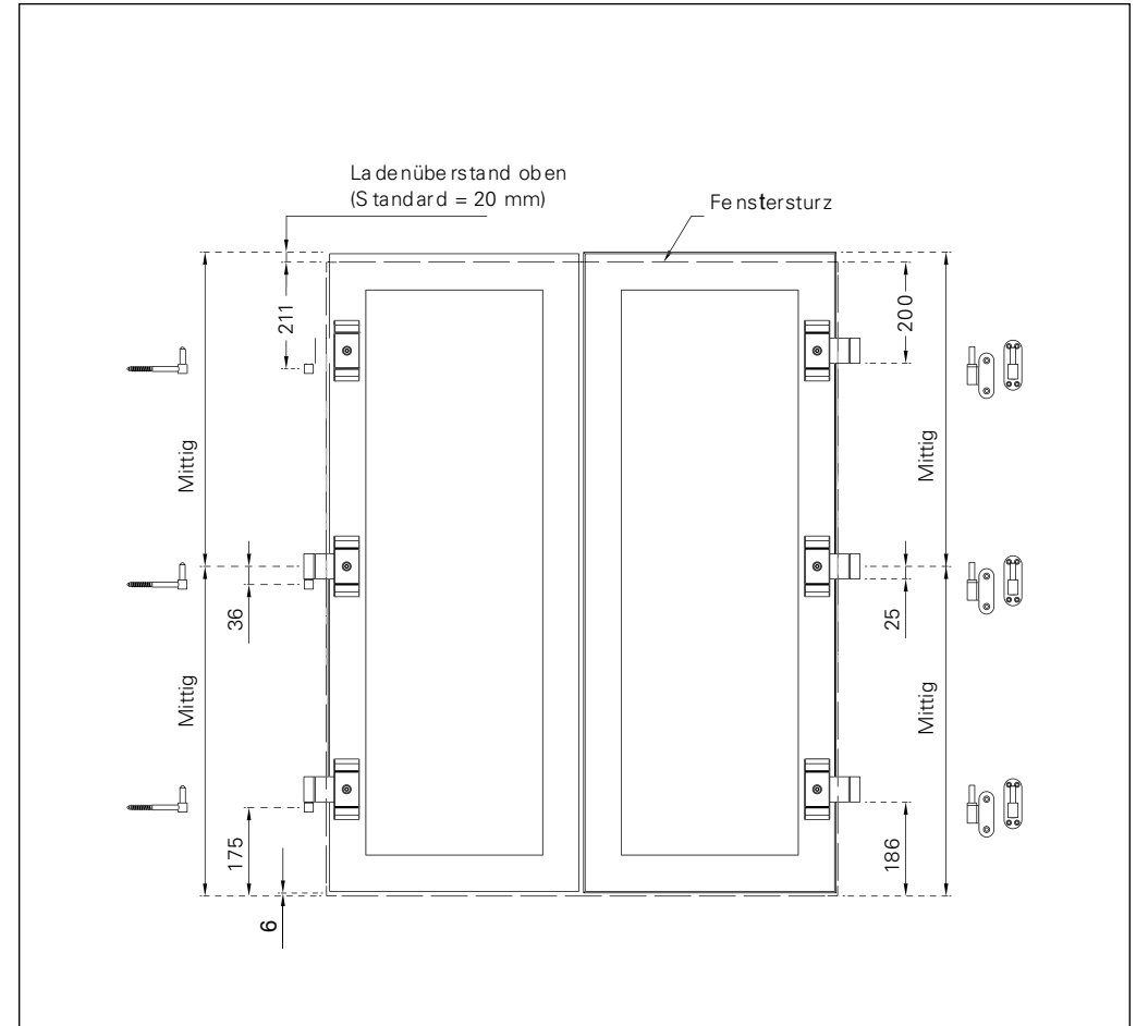
Montageart 4
