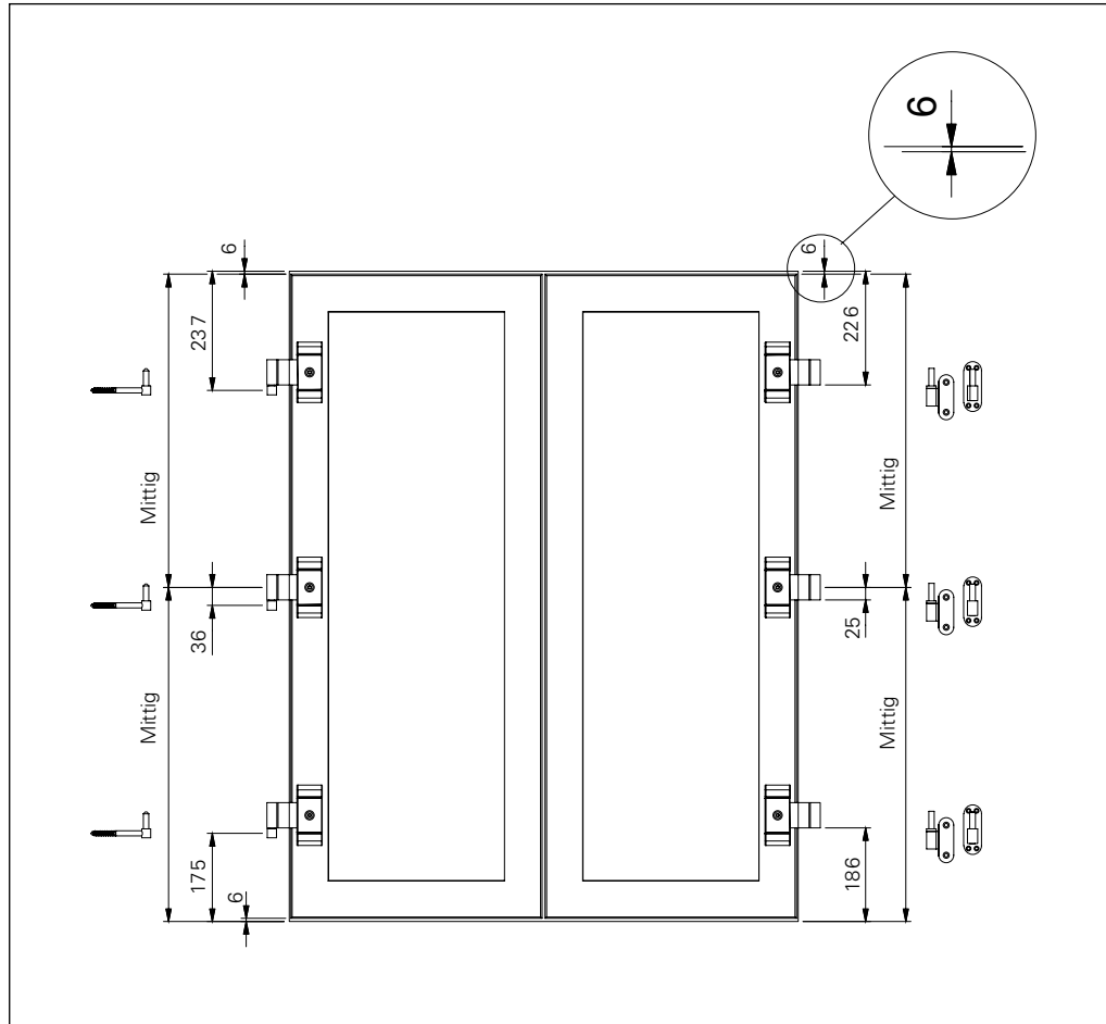
Montageart 1, 2, 3
