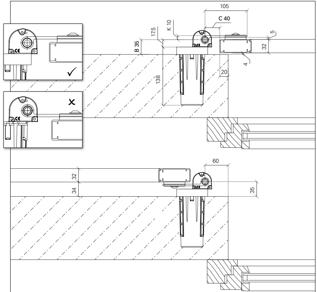
Montageart 4 aufliegend
