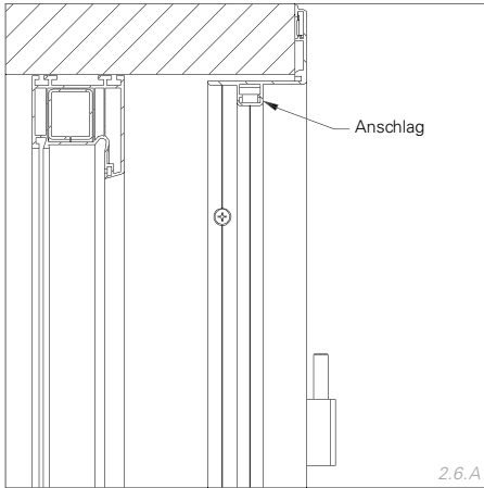
Variante A Zarge befestigen hinter Anschlag
