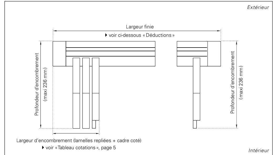
Coupe horizontal
