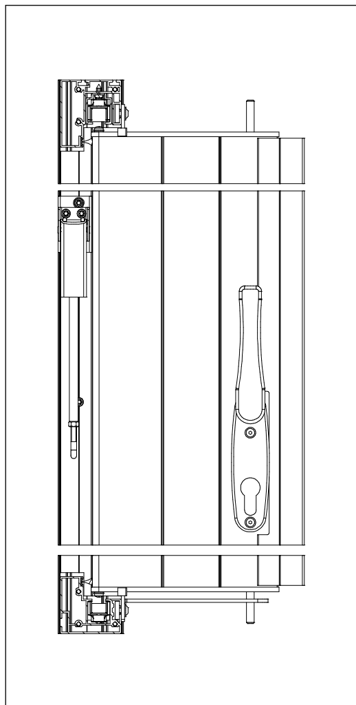
Coupe vertical
