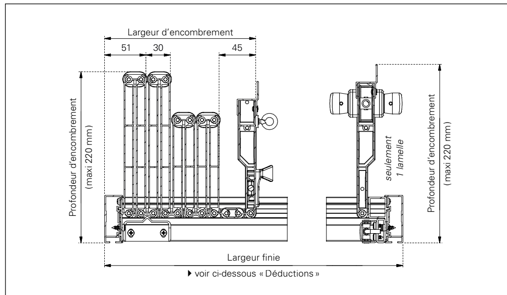
Coupe horizontal
