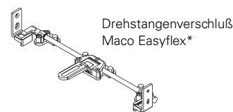
+ T-Leiste + Zuziehgriff* + Verriegelungswinkel*
