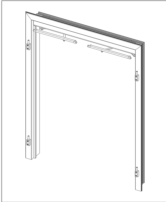
Bastidor rápido Z135 + VOLETRONIC
