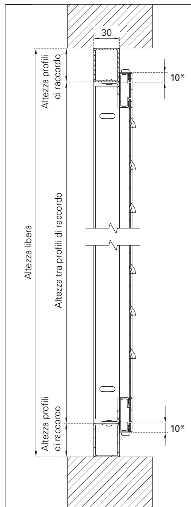
Profilo di raccordo in alto e in basso
