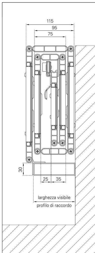
Sezione del sistema
