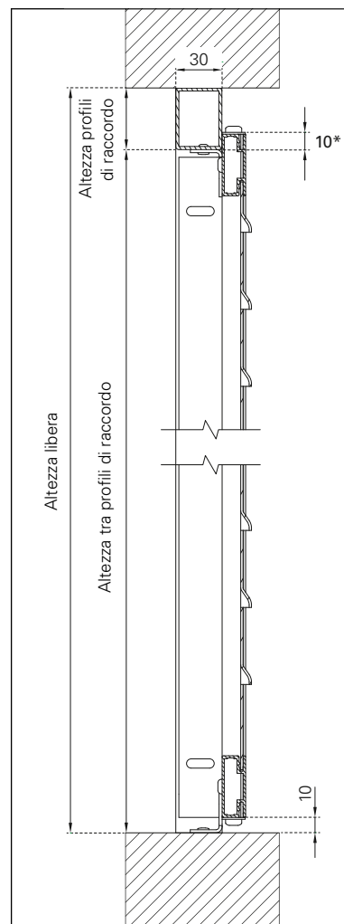
Profilo di raccordo solo in alto
