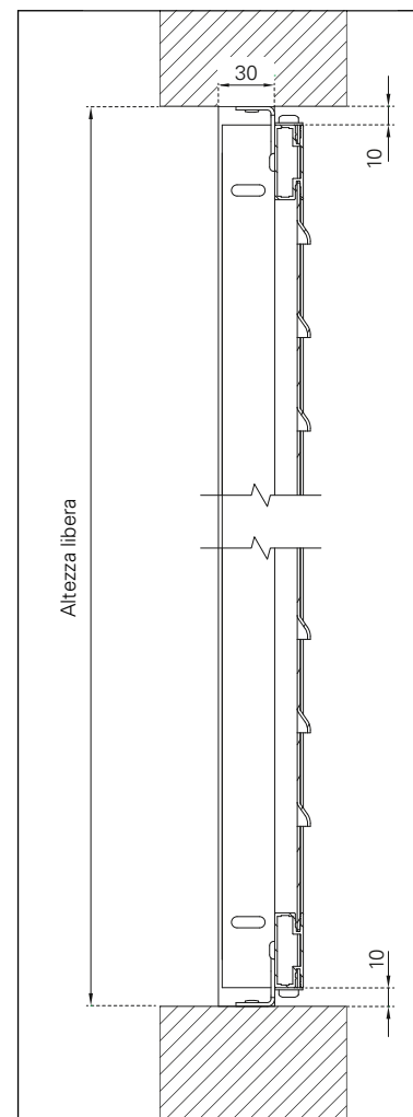
Senza profilo di raccordo
