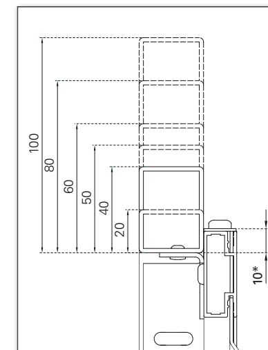
Altezze del profilo di raccordo
