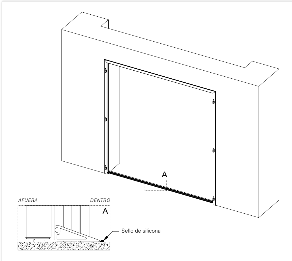
Bastidor montado desde fuera / abriendo hacia afuera
