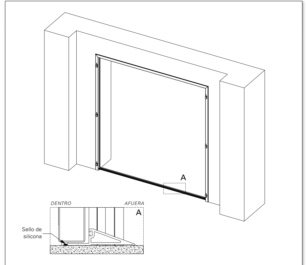
Bastidor montado desde dentro / abriendo hacia adentro
