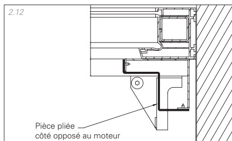
Pièce pliée côté opposé au moteur
