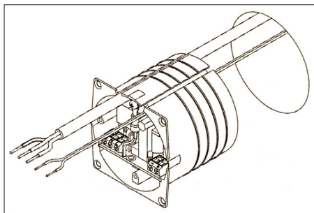
Inserimento cavi
