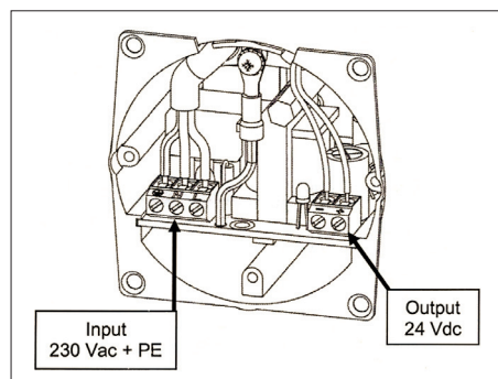
Collegamento elettrico
