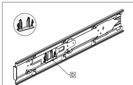
Dettaglio del coperchio laterale
