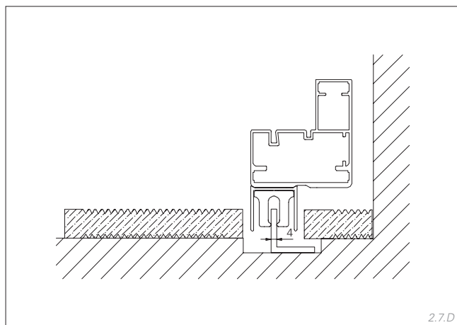
Guida a terra Tipo D per l'installazione in sito su una base solida. Non vi è alcun aggiustamento in fase di installazione Tipo D.
