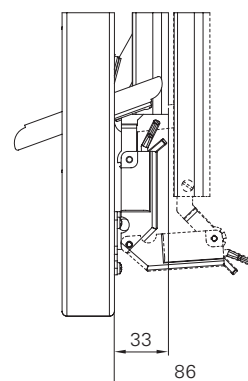
Verstellhebel
