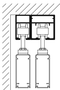
Exemple : 2 rails avec cadre R75
