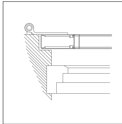
Montage 3 pose entre feuillure
