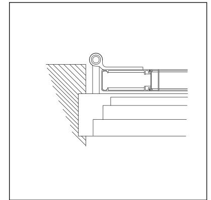
Montage 5 pose sur dormant
