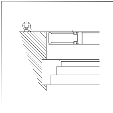
Montage 1 pose entre tableau
