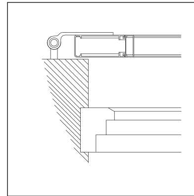
Montage 4 pose en applique
