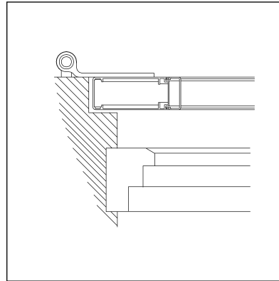
Tipo di montaggio 3
