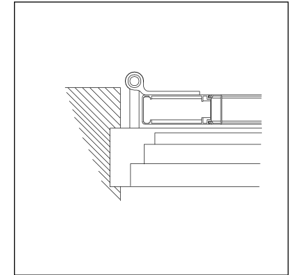
Tipo di montaggio 5
