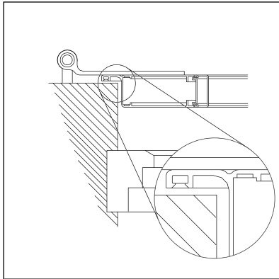
Tipo di montaggio 2 con battuta
