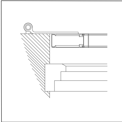
Tipo di montaggio 1
