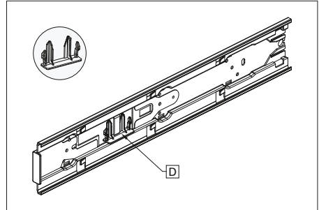
Detail Seitendeckel
