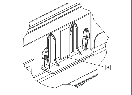
Detail Seitendeckel
