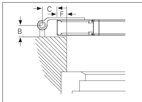
Mode de montage 4 en applique
