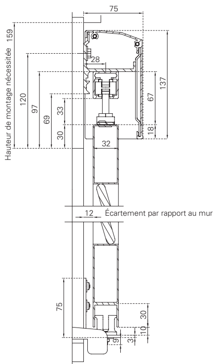
Système A75/60 BT32 | Type A
